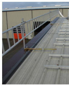
Blechedach-Ortgangsicherung
