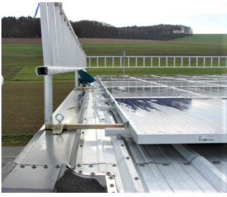
Blechedach-Ortgangsicherung
