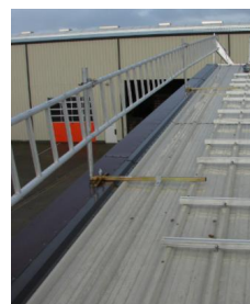
Blechdach-Ortgangsicherung
