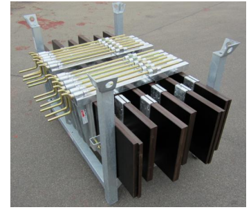
Schalungs-Sortimente
