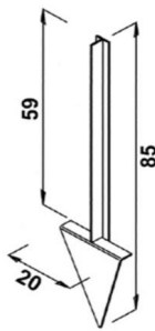
Schnurgerüst Easy Eck
