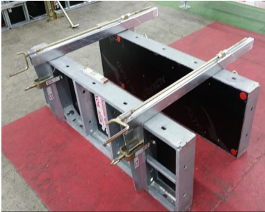
Ringgurt-Schalung H50
