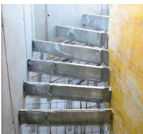
Treppen-Stufen-Schalung
