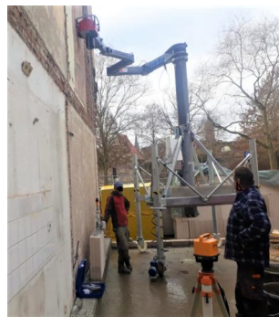
Stein-Rex ® Mauerkran f. Großformat-Steine
